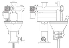
dosatori a coclea
